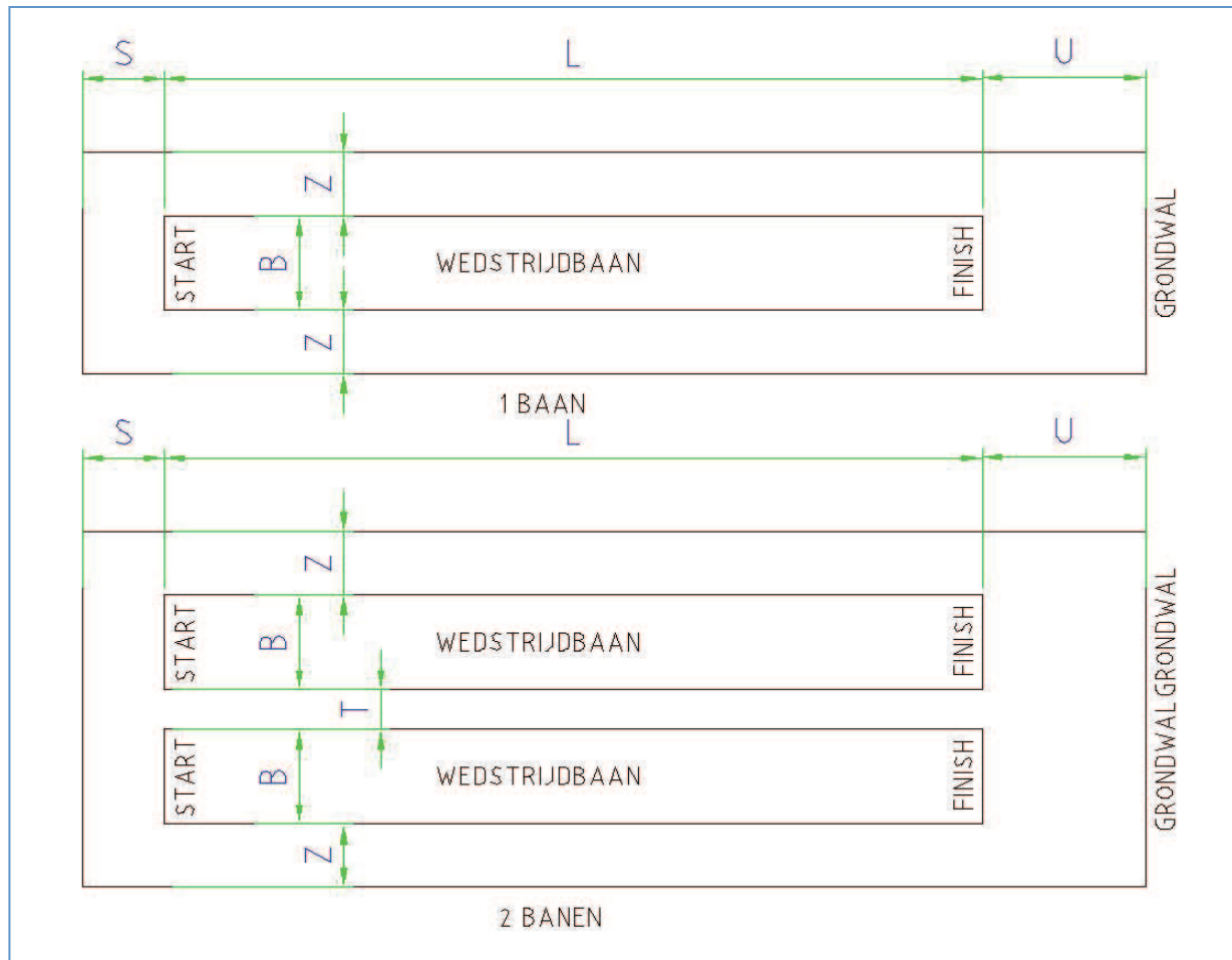
Figuur 1: Baanafmetingen
